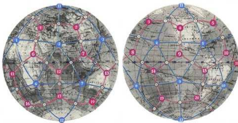
Рис.3 Икосаэдро-додекаэдрическая структура Земли
