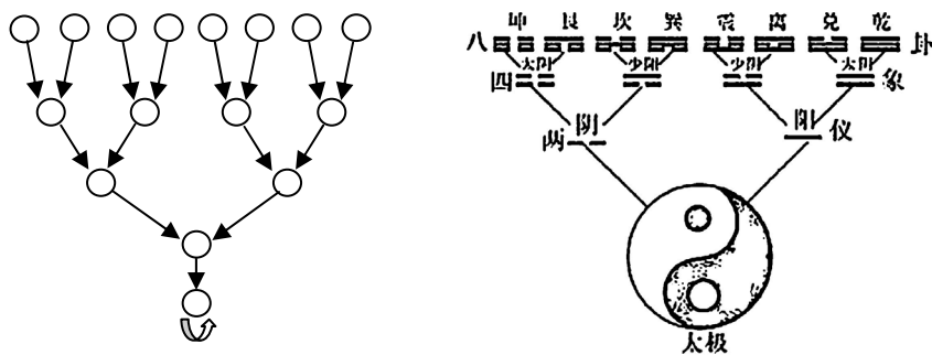
Бинарное древо T_{16} , состоящее из 16 вершин и одного цикла O_1 , и Великий предел «И-цзин».
