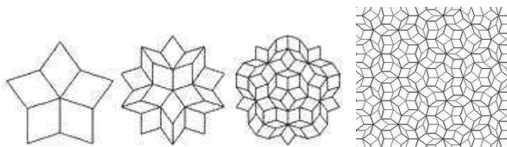
Рис. 1. Структура пентагональных квазикристаллов отвечает объемным (трехмерным) узорам Пенроуза.
