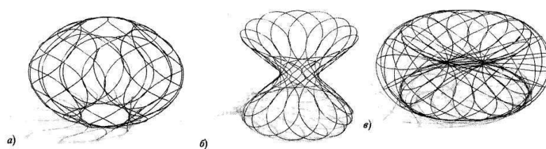
Рис. 5. Примеры NODUS-структур [18]: а) NODUS-структура, моделирующая поверхность эллиптической кривизны; б) та же структура, но вывернутая наизнанку, моделирует поверхность гиперболической кривизны; в) модель тора как комбинация фрагментов поверхностей эллиптической и гиперболической
