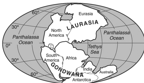
Разделение единого сверхконтинента Пангеи на Лавразию и Гондвану.
